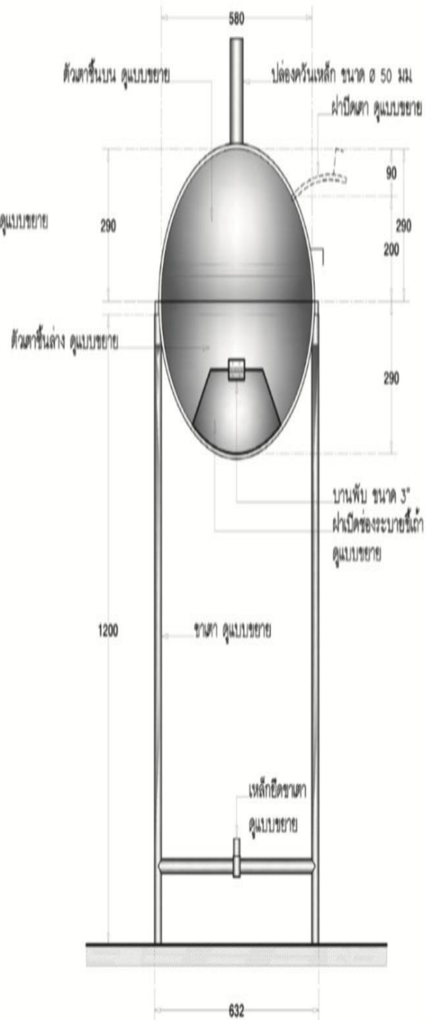
รูปตั้งด้านข้าง มาตราส่วน 1:12.5
