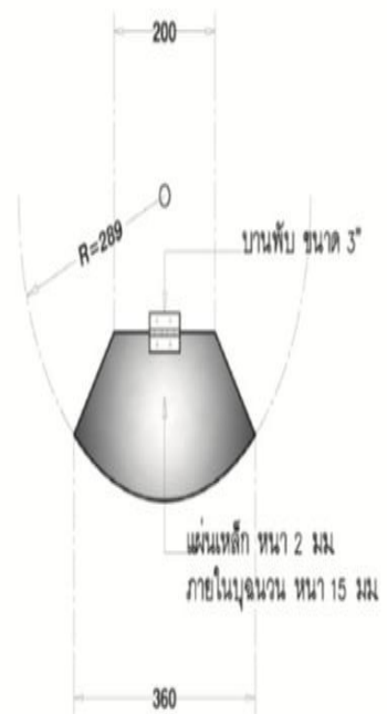
แบบขยายฝาปิดช่องระบายน้ำ มาตราส่วน 1:10
