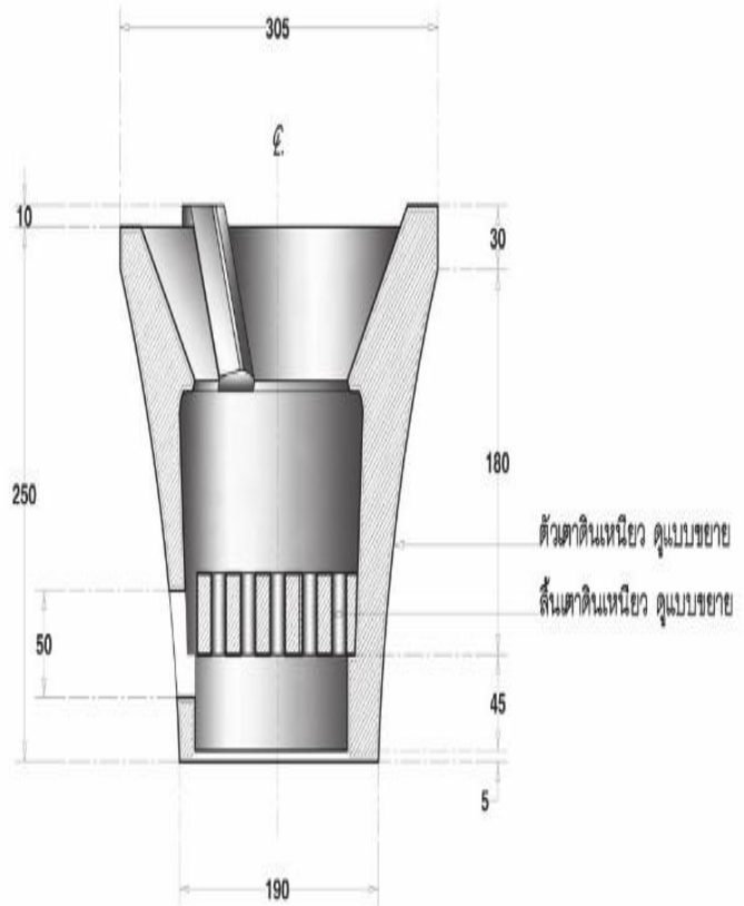
รูปตัด B มาตราส่วน 1:5
