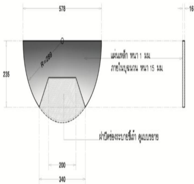
แบบขยายฝาดังด้านข้าง มาตราส่วน 1:10
