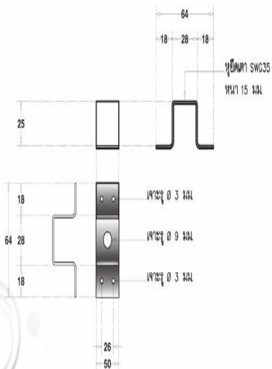
แบบขยายรูยึด มาตราส่วน 1:2.5
