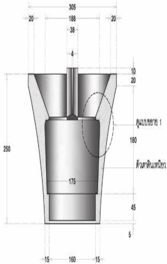
รูปตัด A มาตราส่วน 1:5
