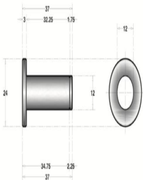
แบบขยายสลัก ขนาดส่วน 1:1
