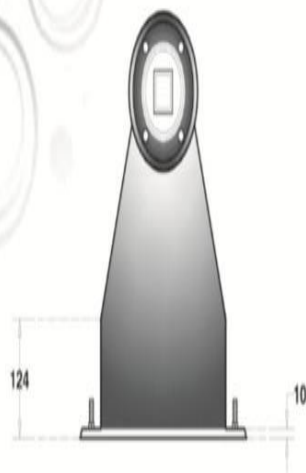
รูปตัดด้านหน้า มาตราส่วน 1:10
