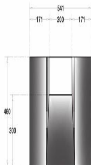
รูปตั้งด้านหลัง
