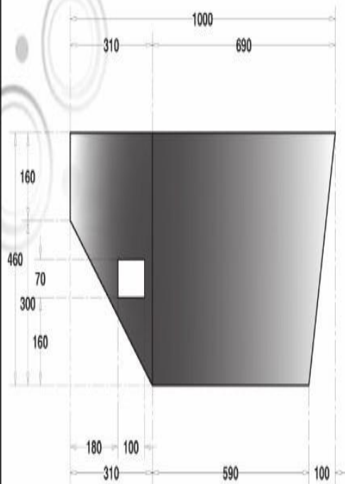
รูปตั้งด้านข้าง
