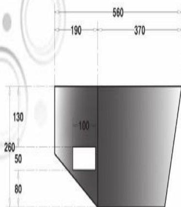
รูปตั้งด้านข้าง
