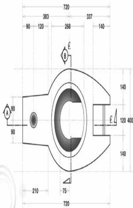
แบบขยายเตาเศรษฐกิจขนาดกลาง
