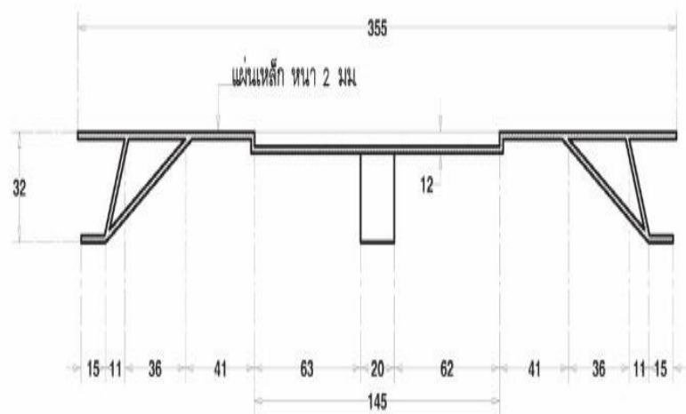
แบบขยายขาตั้งเตา
