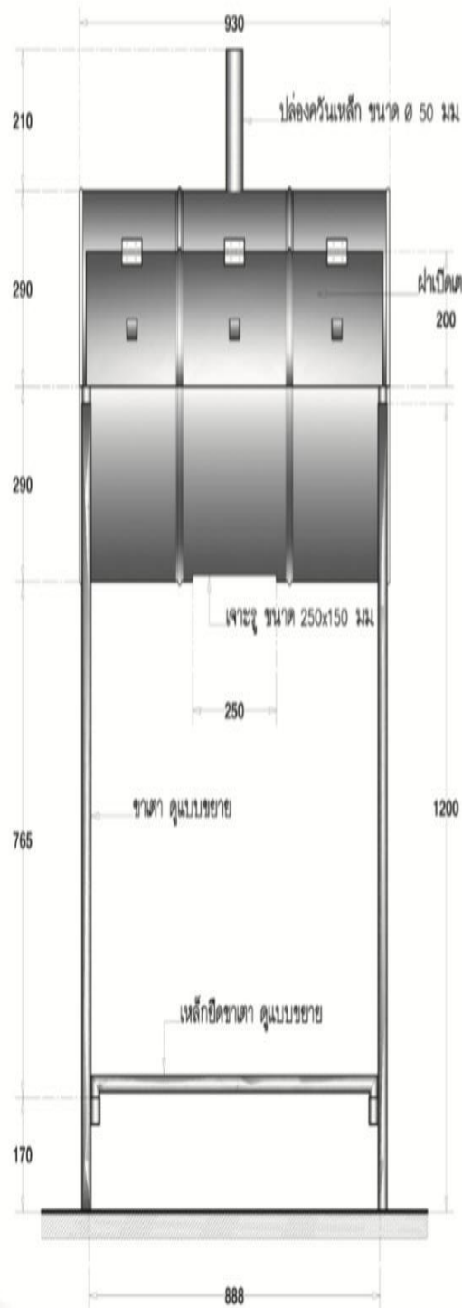
รูปตั้งด้านหน้า มาตราส่วน 1:12.5
