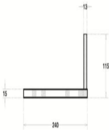
รูปตัดด้านหน้า มาตราส่วน 1:5
