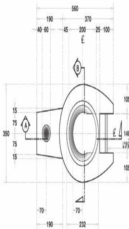
แบบขยายตาเศรษฐกิจขนาดเล็ก
