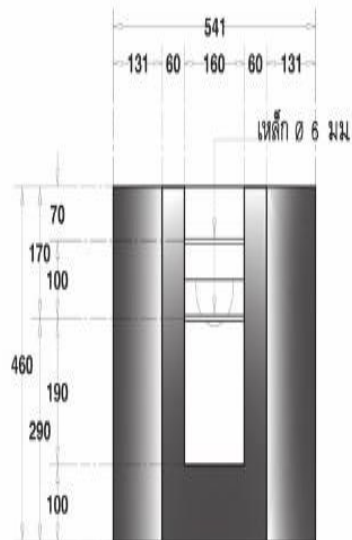
รูปตั้งด้านหน้า
