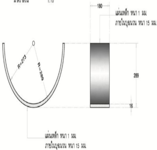
แบบขยายจนจนกันความร้อนด้านใน มาตราส่วน 1:10
