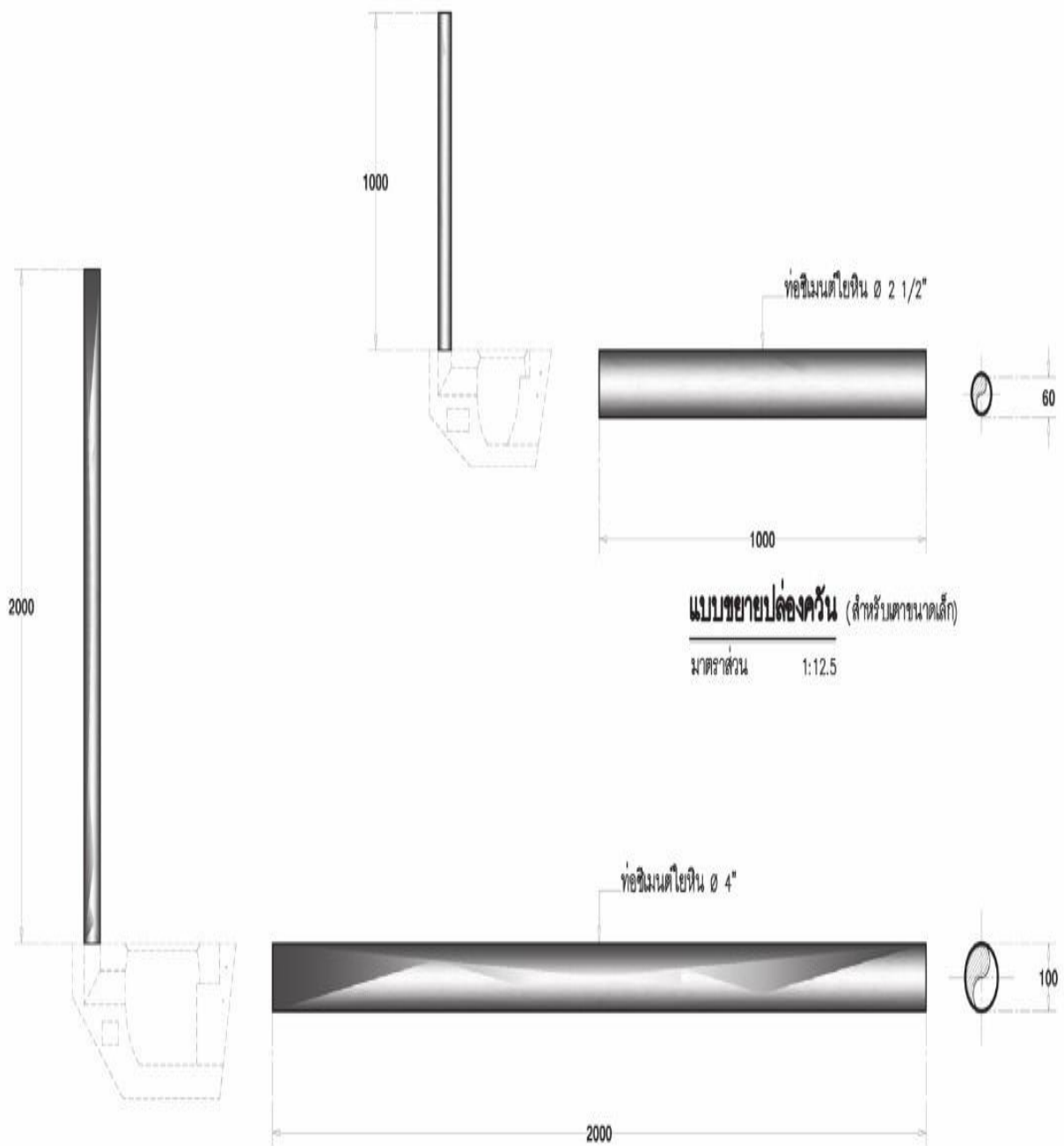
แบบขยายปล่องคว้น (สำหรับเตาขนาดกลางและใหญ่) มาตราส่วน 1:12.5
