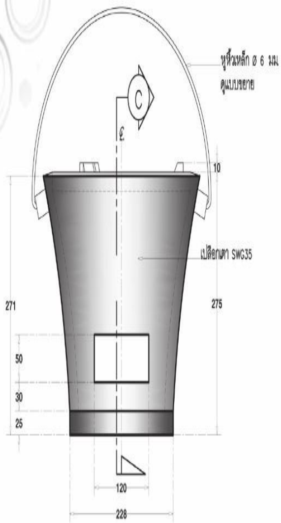
แบบขยายเปิดอกตา มาตราส่วน 1:5
