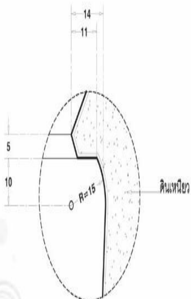
แบบขยาย 1 มาตราส่วน 1:5
