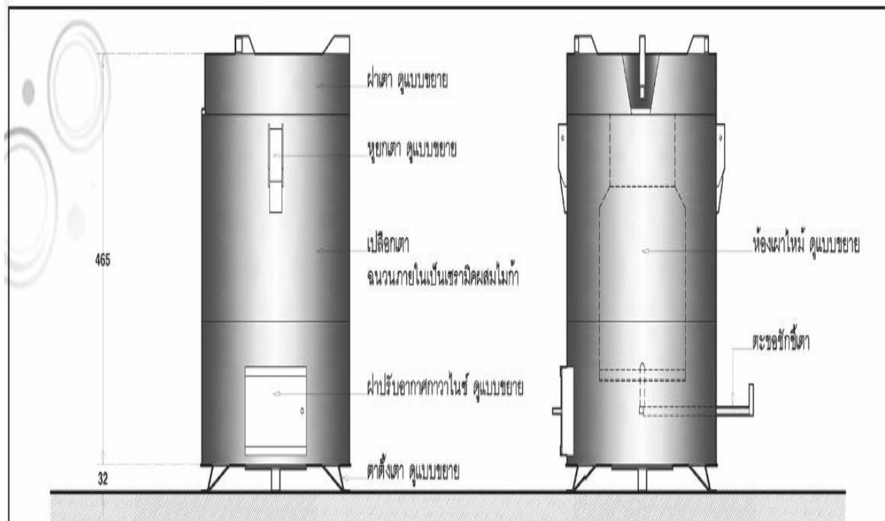
รูปตั้งด้านหน้า
