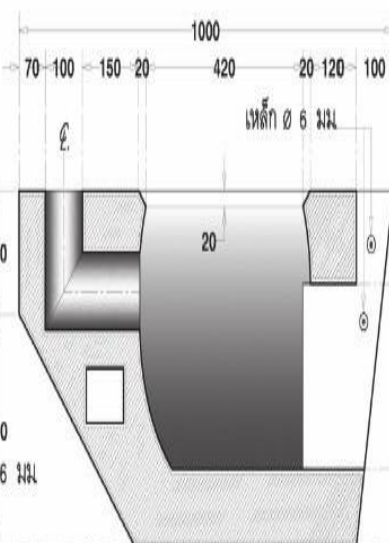
รูปตัด A
