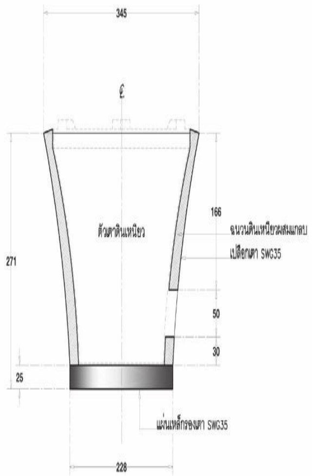
รูปตัด C มาตราส่วน 1:5
