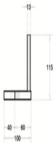
รูปตัดด้านข้าง มาตราส่วน 1:5
